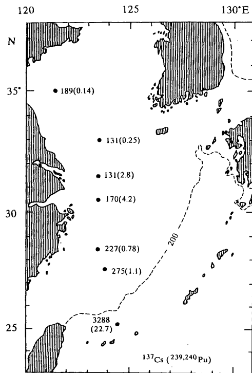
図 2. 海水中(表面~海底)の ^{137}\text{Cs} および ^{239,240}\text{Pu} 全量(MBq/km 2 )
