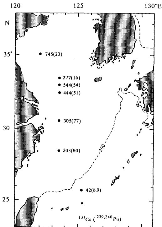
図 3. 海底堆積物中(0~20cm)の ^{137}\text{Cs} および ^{239,240}\text{Pu} 全量(MBq/km 2 )
