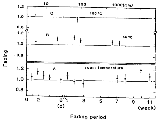
図2 室温照射した蔗糖内遊離基のフェーディング。 A: 室温保存, B: 55°C, C: 100°C保存
